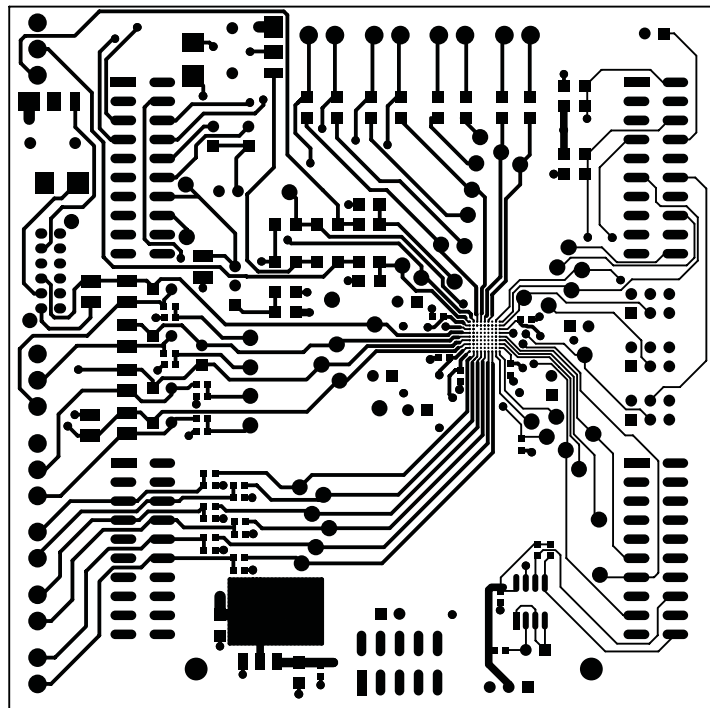
Figure C-2. Top Layer
